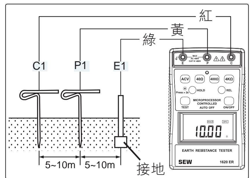
接地電阻量測
